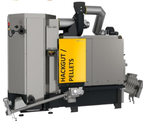
ETA HACK VR Hackgutkessel mit Vorschubrost 250 bis 500 kW
